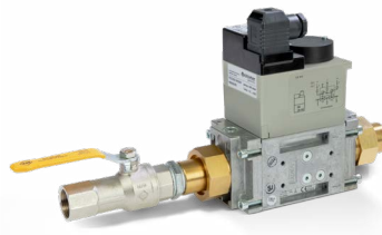
GASABSPERREINRICHTUNG FSA 320
