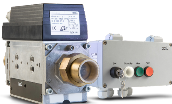
SCHALKASTEN SK 32
