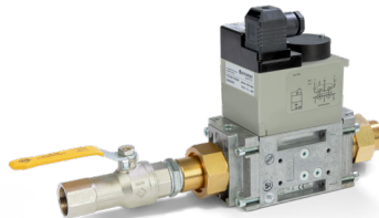
GASABSPERREINRICHTUNG FSA 320
